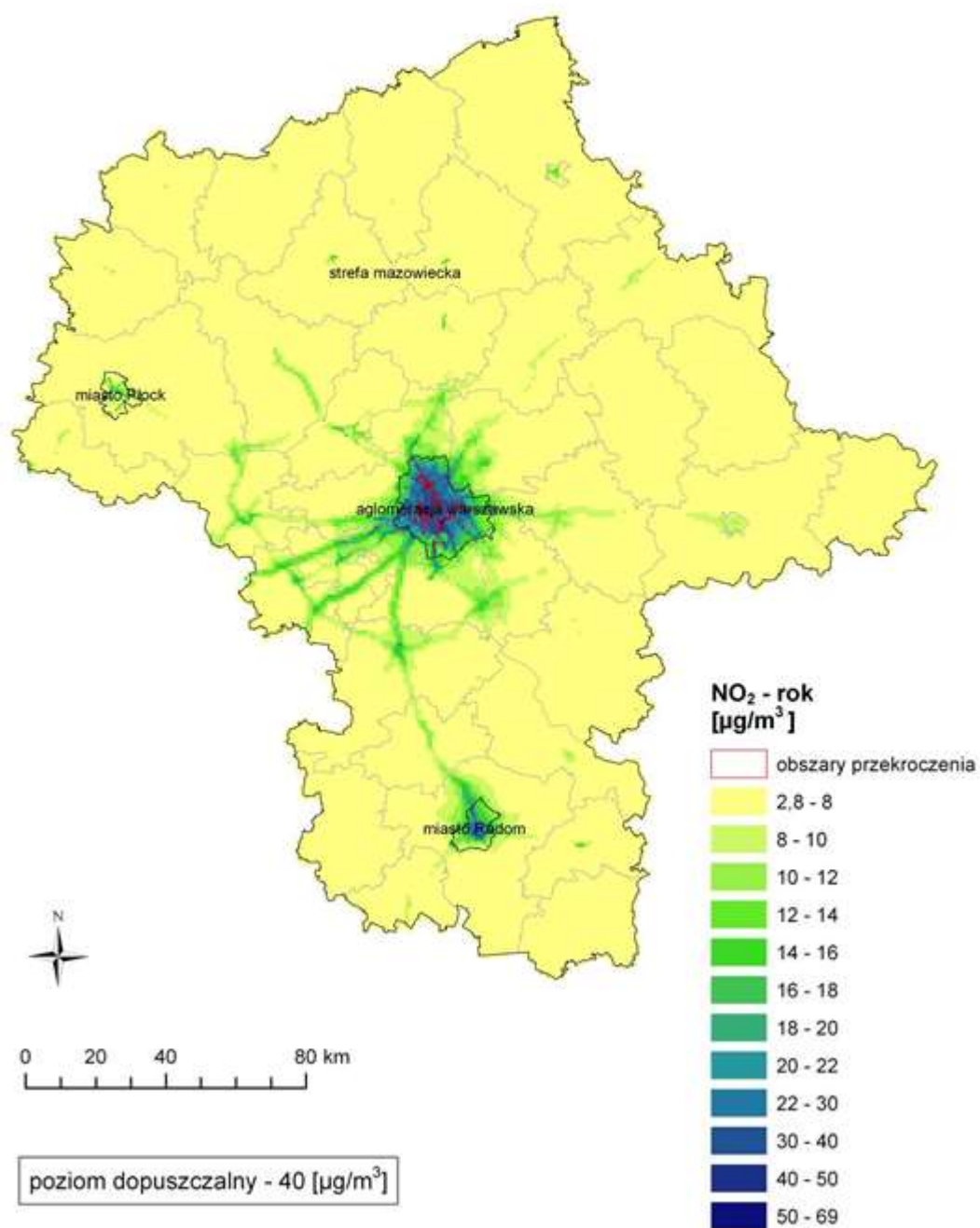
Mapa 2.1. Rozkład stężeń \text{NO}_2 -rok na obszarze województwa mazowieckiego (rok 2015) (źródło: WIOŚ w Warszawie)
