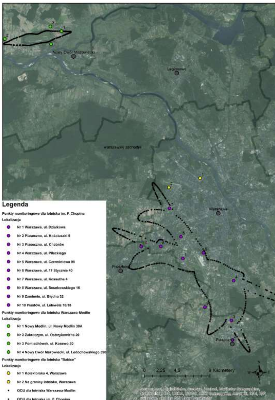
Mapa 4.2. Lokalizacja punktów monitoringowych dla hałasu lotniczego oraz obszarów ograniczonego użytkowania wokół lotnisk (źródło: WIOŚ, Port Lotniczy im. F. Chopina, Port Lotniczy Warszawa-Modlin oraz uchwały Sejmiku Województwa Mazowieckiego)
