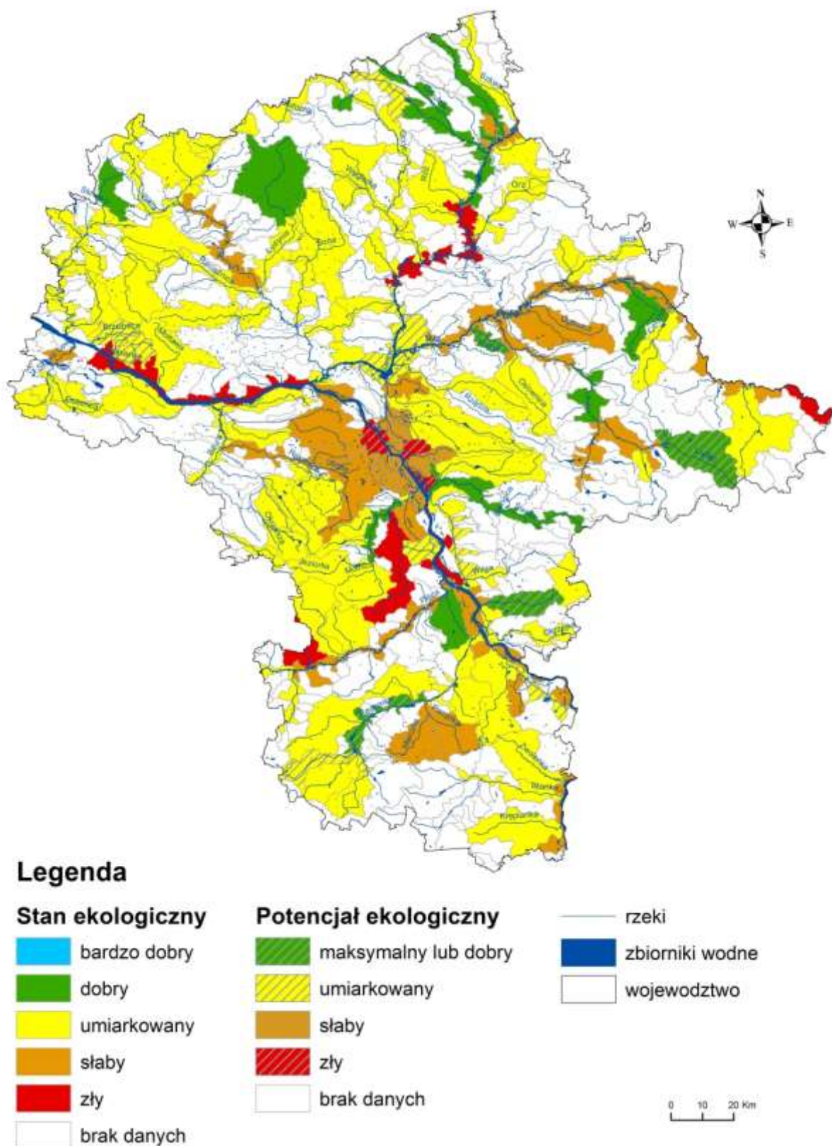
Mapa 3.1. Wyniki oceny stanu/potencjału ekologicznego JCWP rzecznych województwa mazowieckiego za okres 2010-2015 (źródło: WIOŚ)
