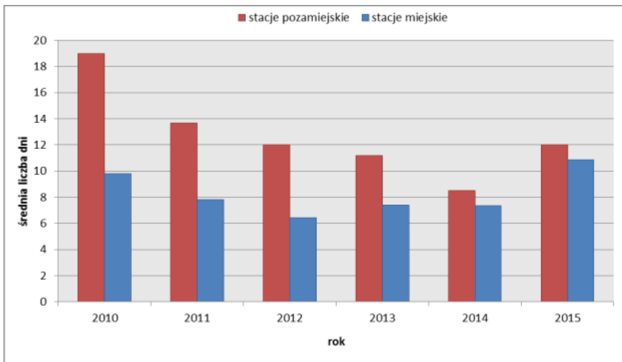
Wykres 2.14. Średnia arytmetyczna z liczby dni ze stężeniami 8-godz. ozonu wyższymi od 120 µg/m³ w latach 2010-2015 w województwie mazowieckim (źródło: WIOŚ w Warszawie)
