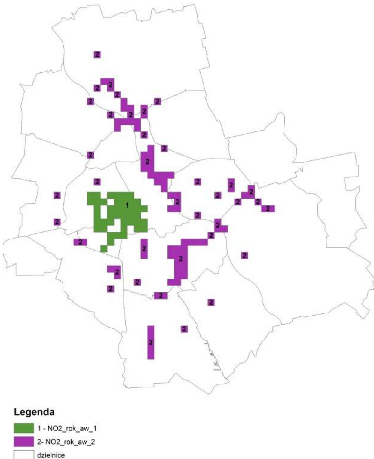
Mapa 2.10. Obszary przekroczeń poziomu dopuszczalnego NO 2 -rok (2015 r.) (źródło: WIOŚ w Warszawie)
