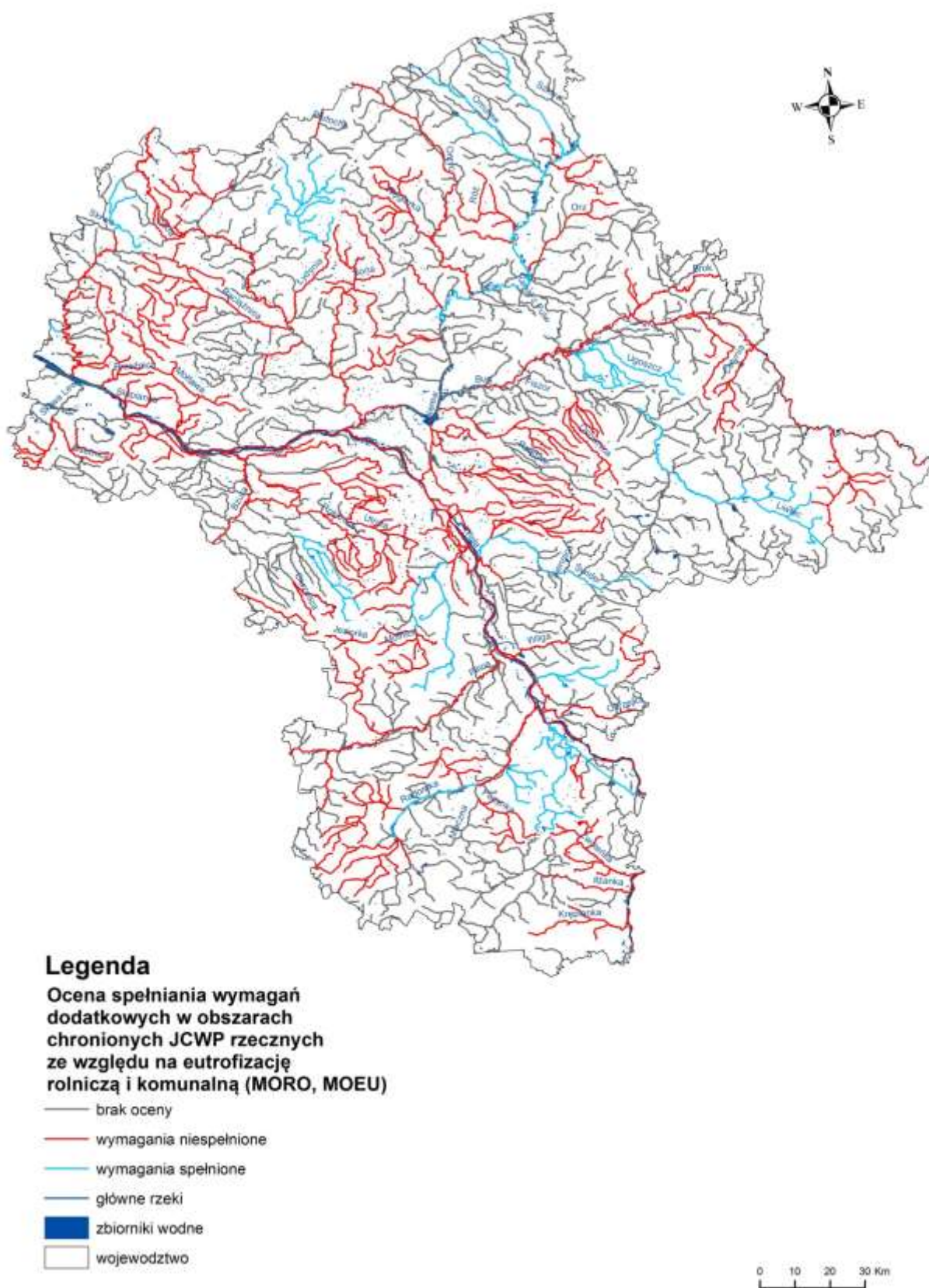
Mapa 3.6. Ocena spełniania wymagań dodatkowych w JCWP rzecznych ze względu na eutrofizację komunalną i rolniczą w latach 2013-2015 (źródło: WIOŚ)
