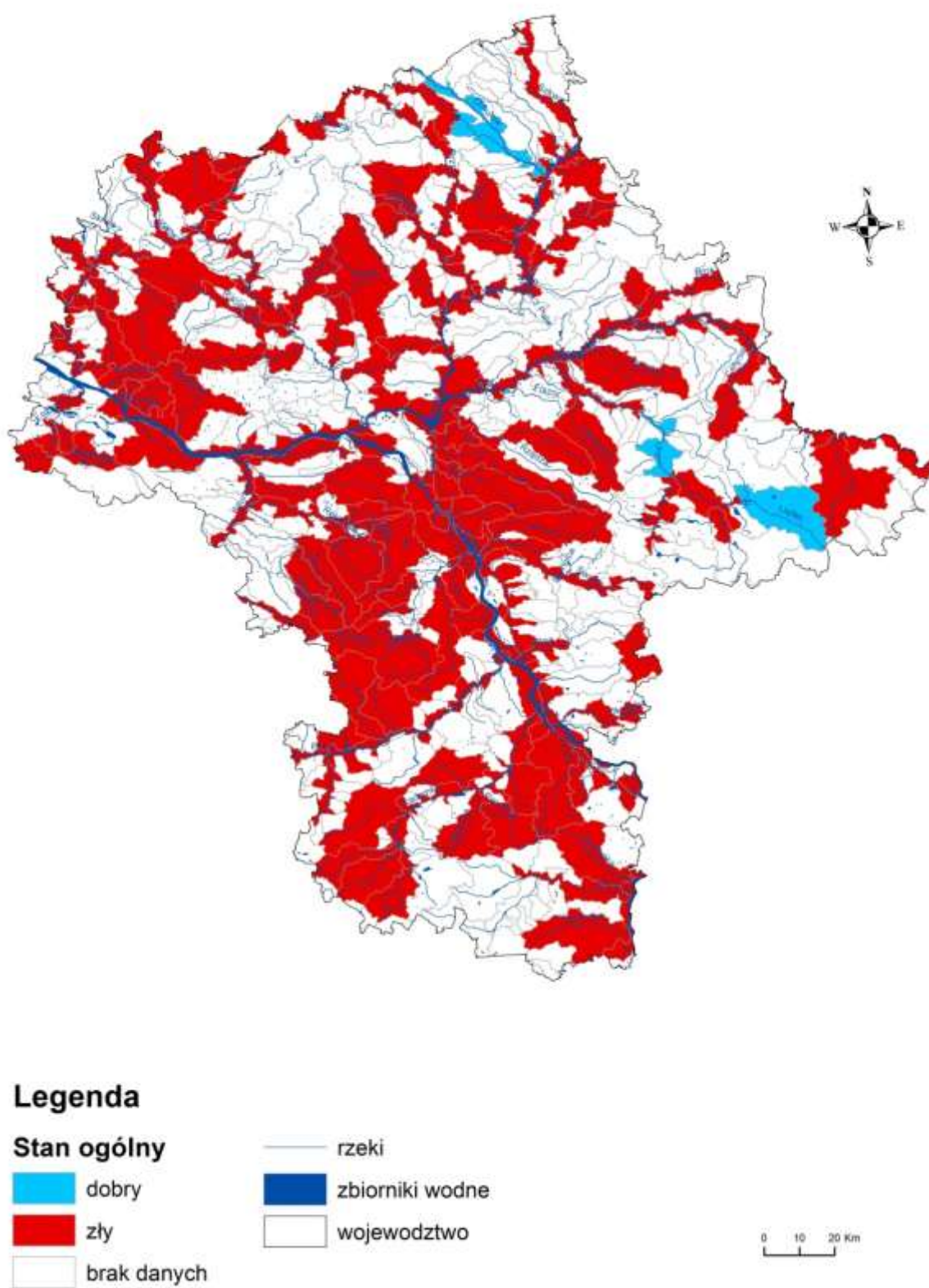
Mapa 3.3. Wyniki oceny stanu JCWP rzecznych województwa mazowieckiego za okres 2010-2015 (źródło: WIOŚ)
