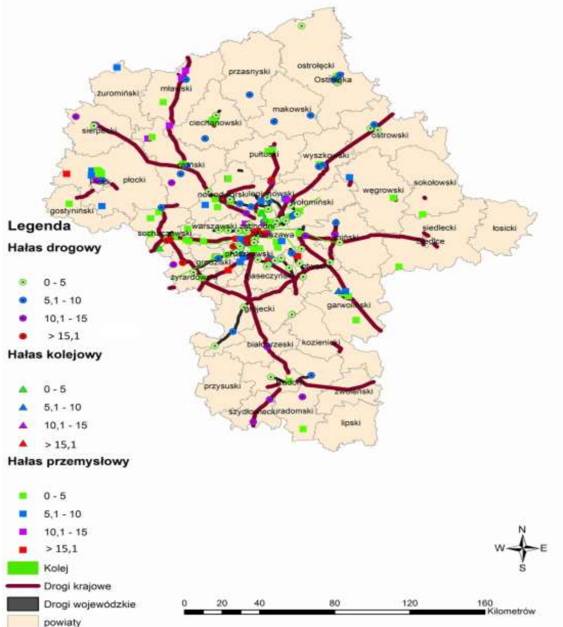
Mapa 4.1. Odcinki dróg oraz torów kolejowych, wzdłuż których wykonano mapy akustyczne oraz przekroczenia poziomów dopuszczalnych hałasu w dB w latach 2013-2015 (źródło: WIOŚ w Warszawie)
